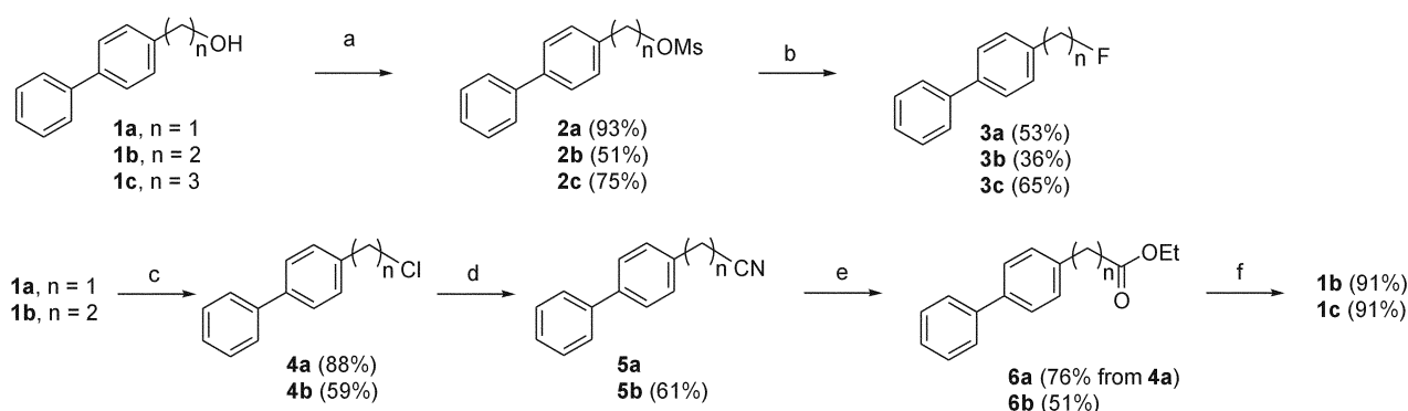
Scheme 2. (a) MsCl, Et 3 N, CH 2 Cl 2 , 0 °C, 30 min; (b) n -Bu 4 NF·xH 2 O, CH 3 CN, 130 °C, 10 min; (c) SOCl 2 , pyridine, benzene, 70 °C, 24 h; (d) NaCN, DMSO, 90 °C, 2 h; (e) CH 3 CH 2 OH, H 2 SO 4 , H 2 O, reflux, 7 h; (f) LAH, THF, -30 °C, 30 min.
