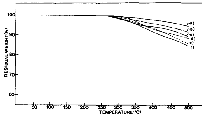
Figure 3. Thermogravimograms of poly(enaryloxynitriles): a) P 16 , b) P 16 , c) P 14 , d) P 6 , e) P 12 and f) P 10 .
